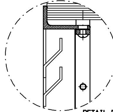
DETAIL D SCHAAL 1:1
