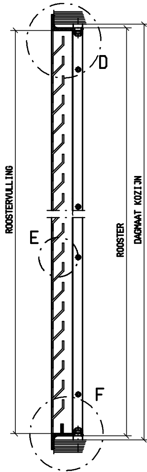
DOORSNEDE schaal 1:2.5
