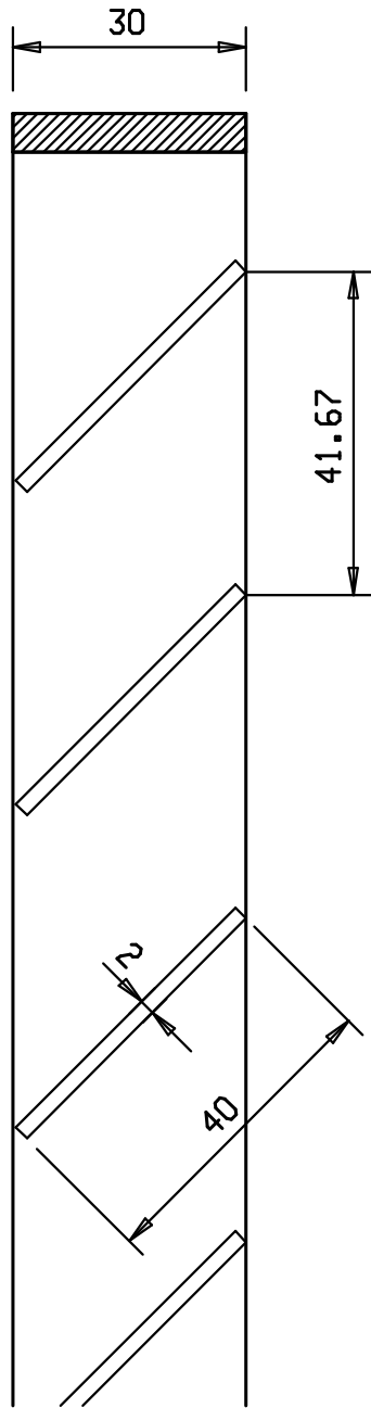
DOORSNEDE B-B
