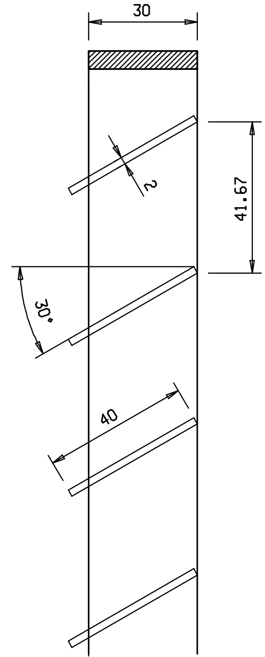
DOORSNEDE B-B
